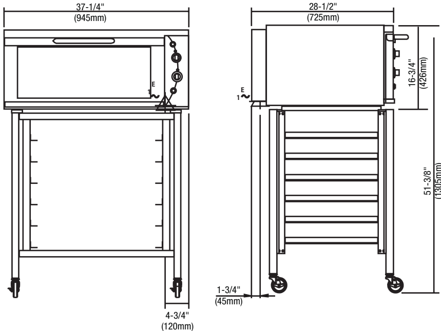
E27MS shown on optional A28CW stand
